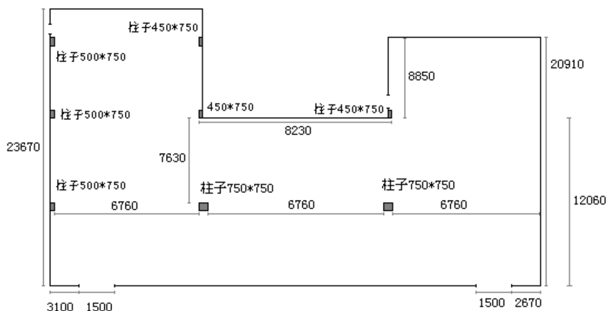
密集库平面图 （单位：mm）
