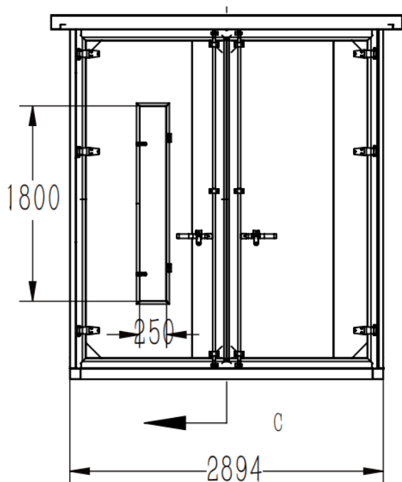
图 4 移动烤房正视图
