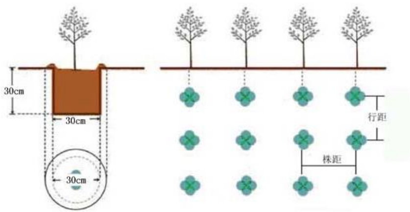
穴状整地栽植模式图
