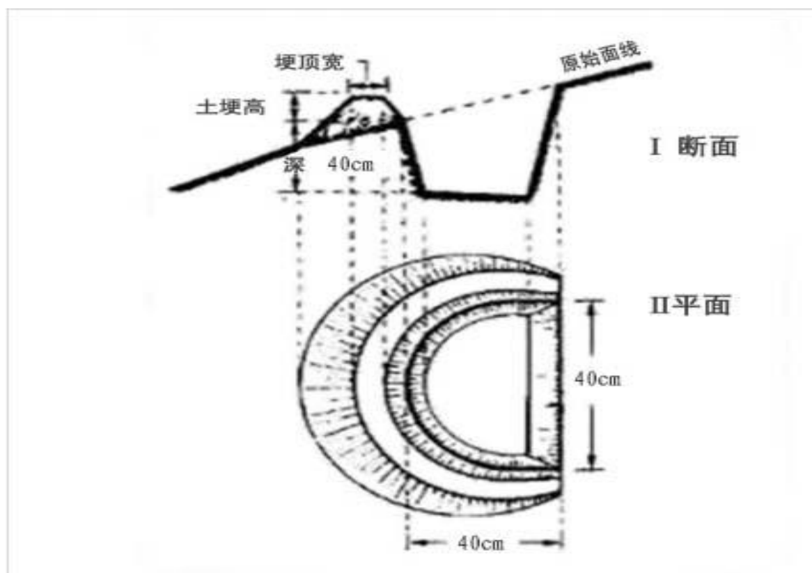
图 5-1 补植补造整地挖穴图式
