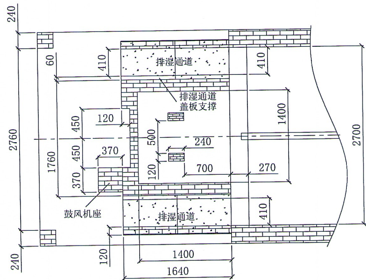
图 5—6 加热室地面俯视图
