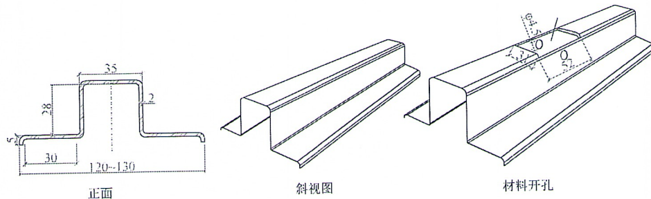
图 5-2 烟梁结构图
