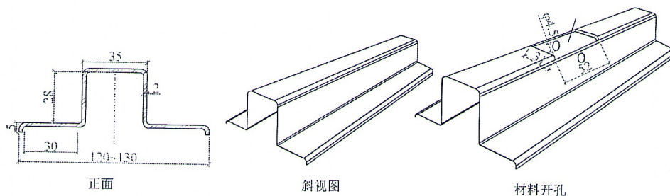
图 5-2 烟梁结构图
