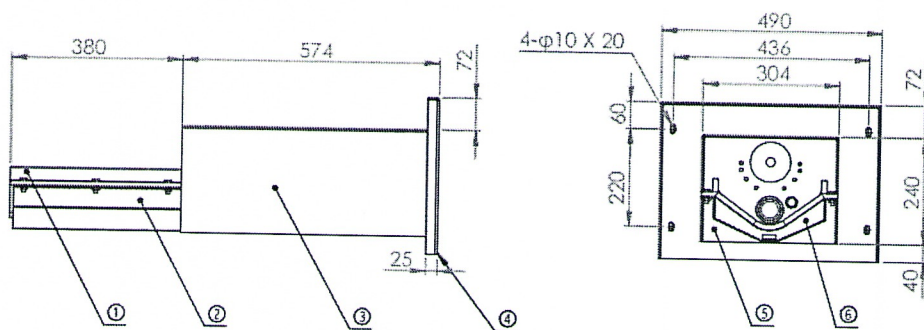
① 燃烧腔；② 燃烧腔底板；③ 配风箱；④ 密封固定板； ⑤ 燃烧弧板挡板；⑥ 燃烧腔底板密封板。
