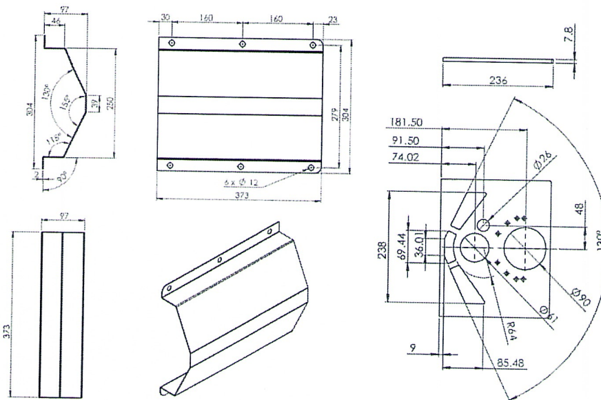
图 9 燃烧弧板底板与燃烧弧板挡板
