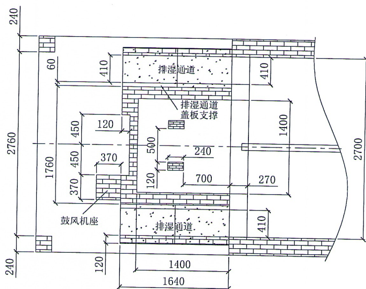
图 5—6 加热室地面俯视图
