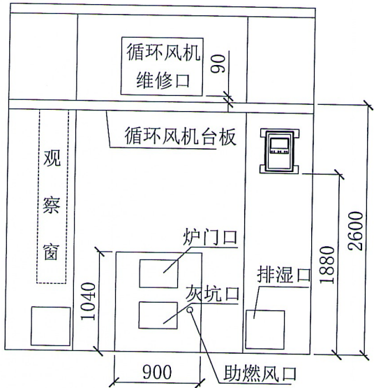
图 5—8 气流下降式前墙
