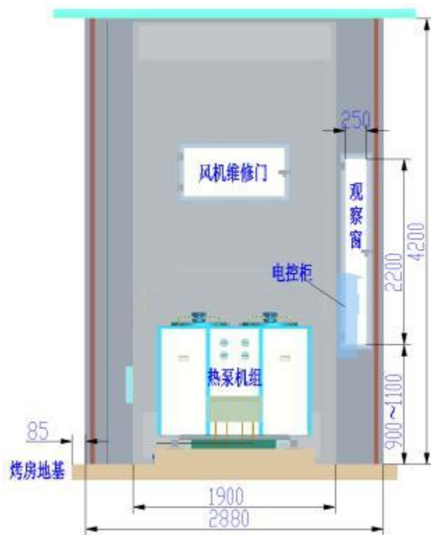
图 3 烤房正视图
