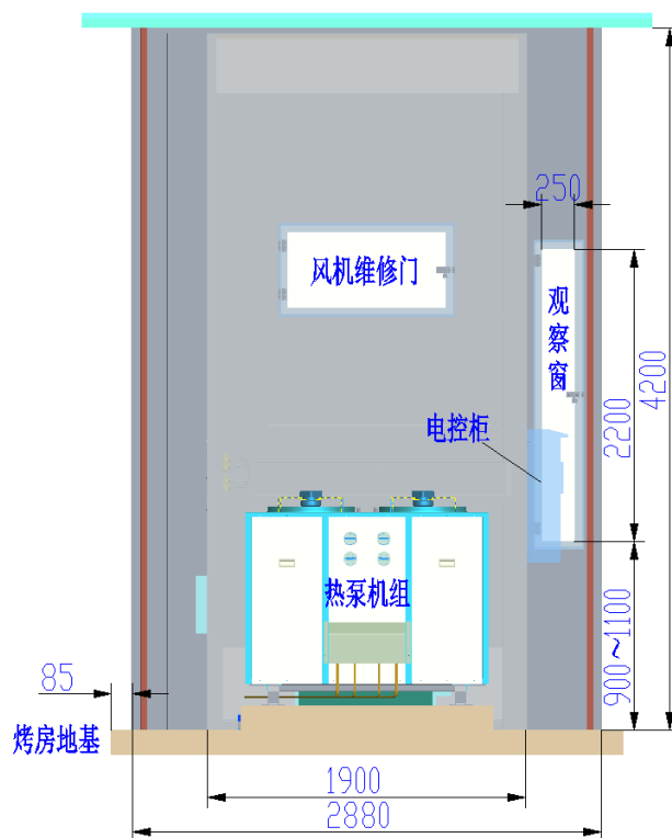
图 3 烤房正视图
