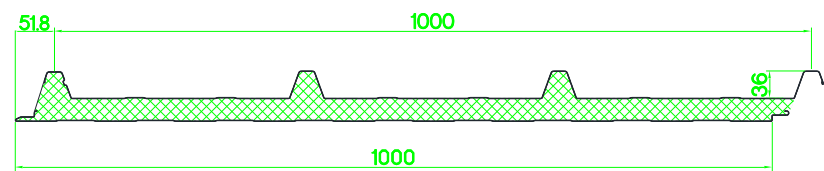
图 5 屋顶板视图
