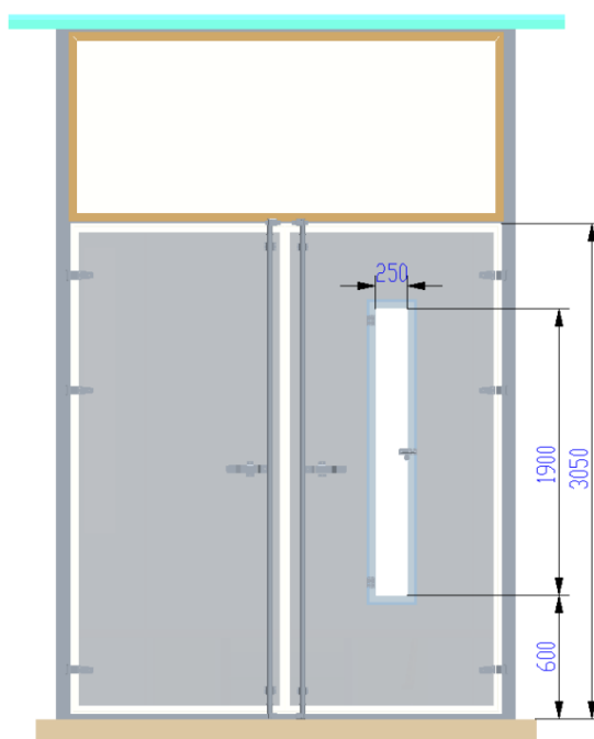
图 8 装烟室大门
