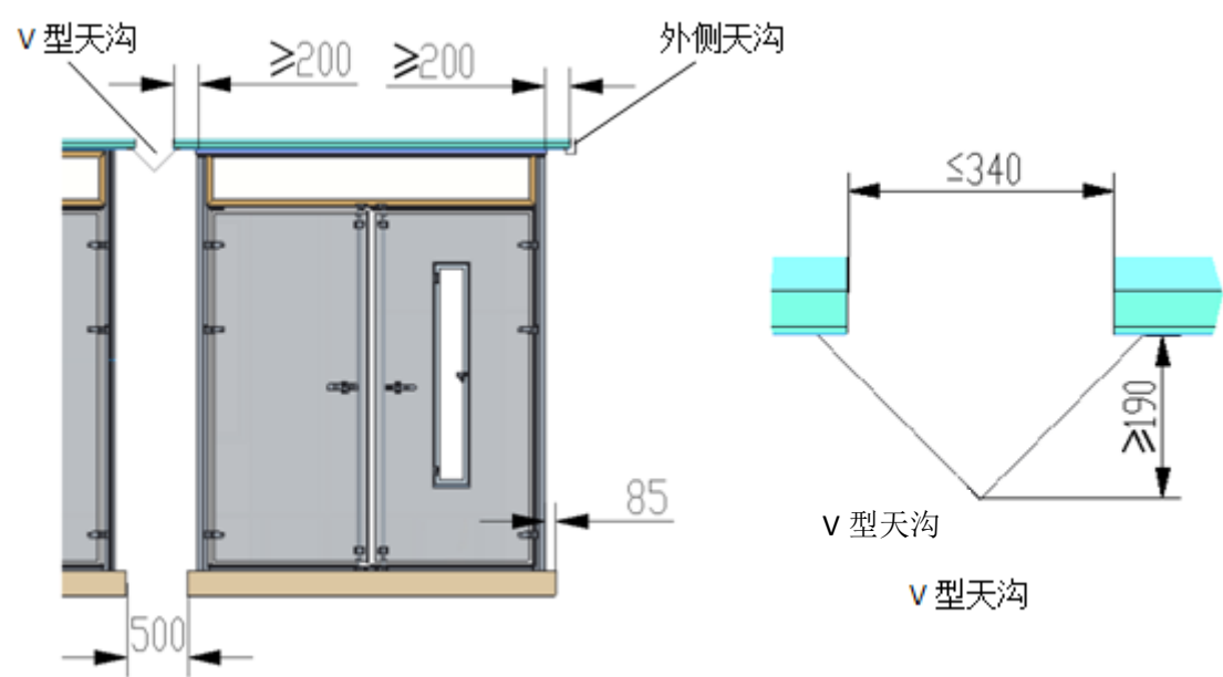
图 6 屋顶板安装要求
