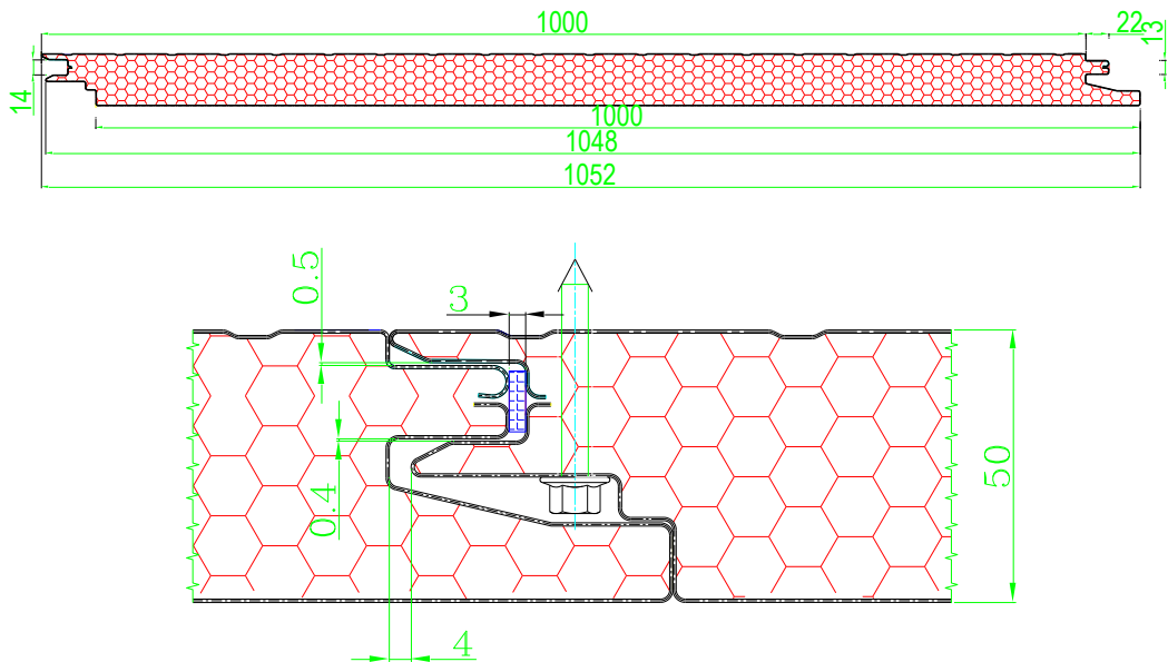
图 4 墙板及连接图
