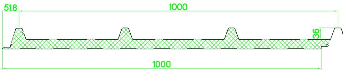
图 5 屋顶板视图
