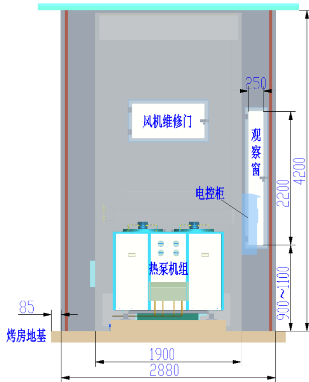
图 3 烤房正视图
