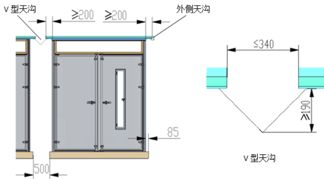
图 6 屋顶板安装要求
