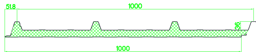
图 5 屋顶板视图
