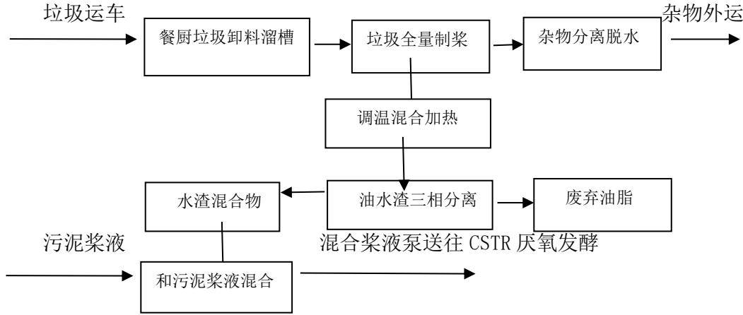
图1：餐厨垃圾预处理工艺流程图
