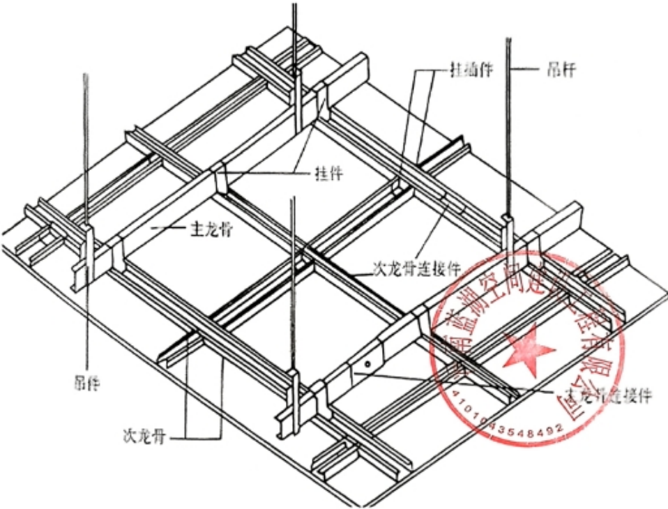
房间吊顶结构图
