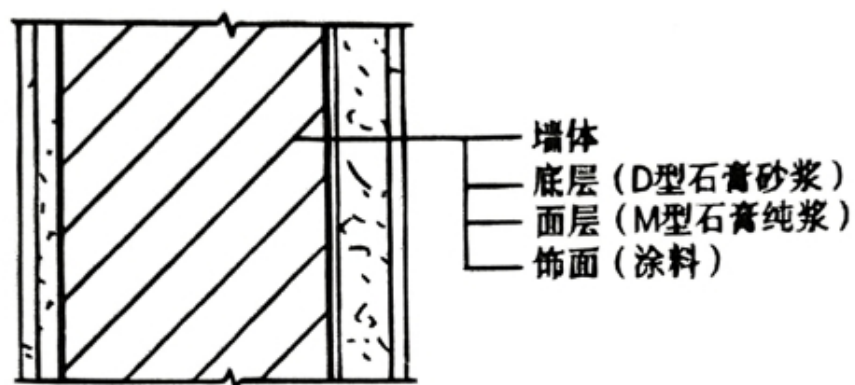
墙面抹灰层构造层次图
