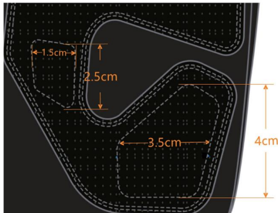
缓冲海绵宽度和高度
