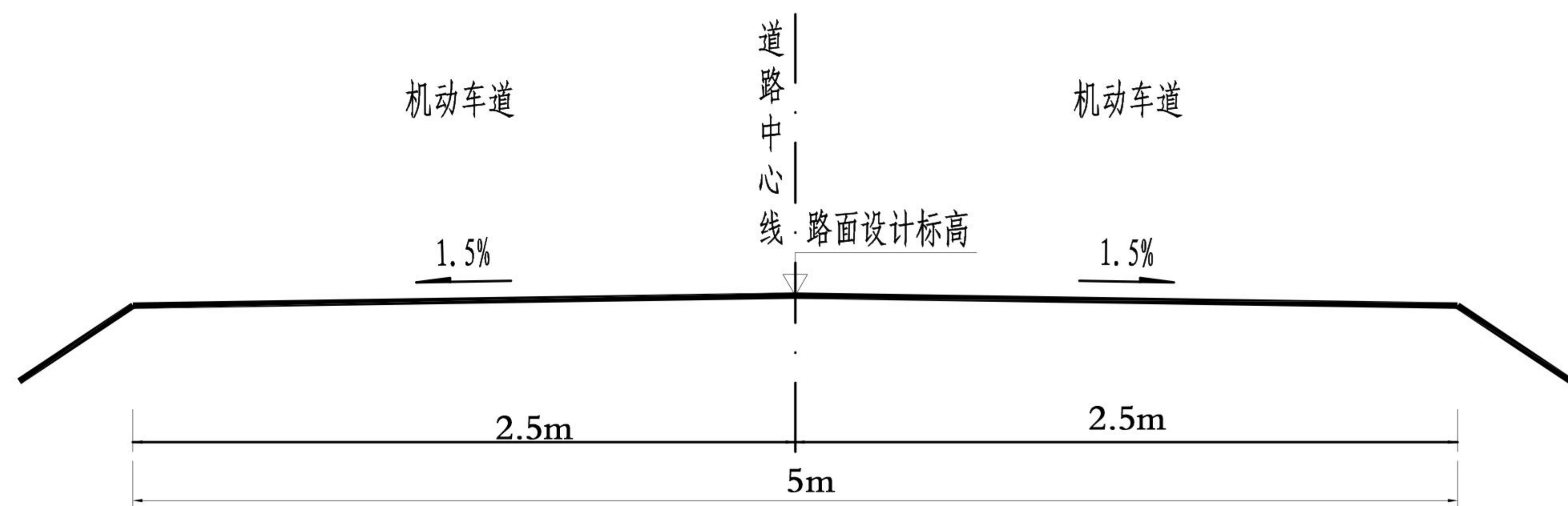
标准横断面图
