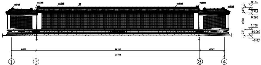
照壁南立面图
