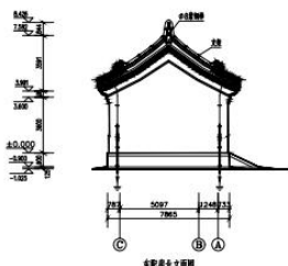
东院大门东立面图
