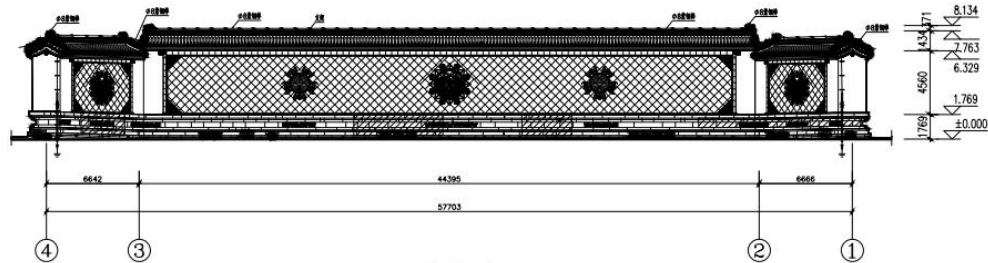
照壁北立面图
