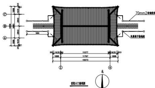
西院大门剖面图
