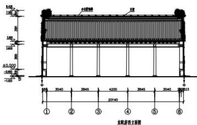
东院大门北立面图
