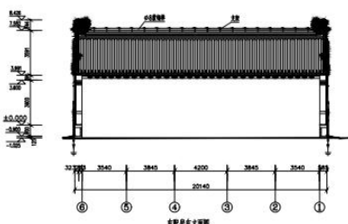
东院大门南立面图
