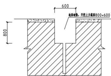
挖沟剖面示意图
