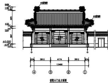
西院大门北立面图
