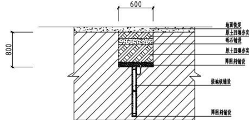
回填剖面示意图
