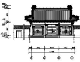
西院大门南立面图
